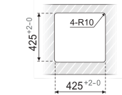
Sobre encimera
